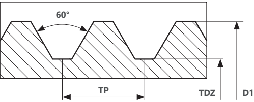
M Метрическая крупная резьба
