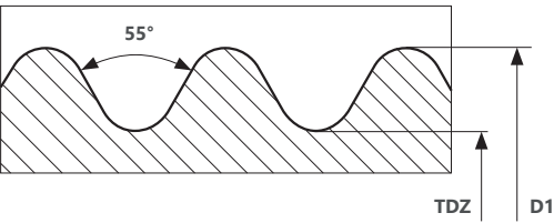
G Трубная резьба
