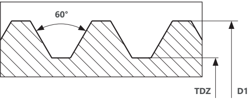
UNC Дюймовая крупная резьба
