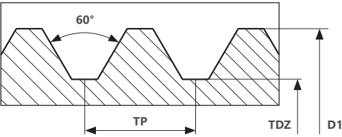
MF Метрическая мелкая резьба
